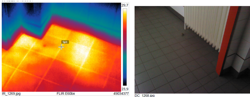
Abbildung 4: Aufnahmen zur Leckageortung
