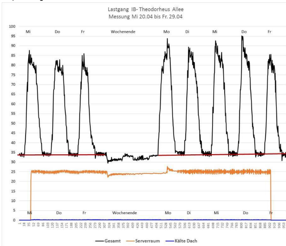
Abbildung 2: Lastgang
