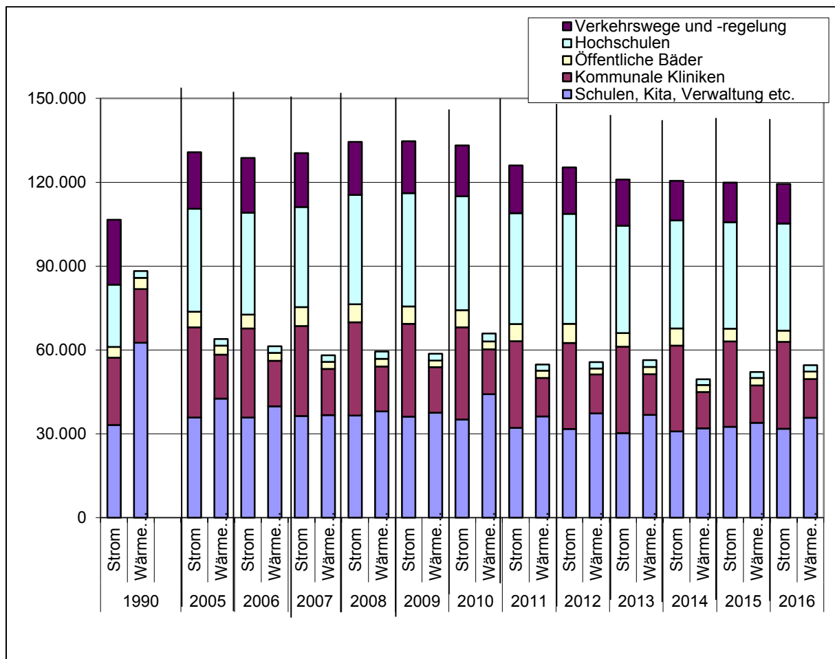
Abbildung 18: CO 2 -Emissionen von 1990-2016 in t/a
